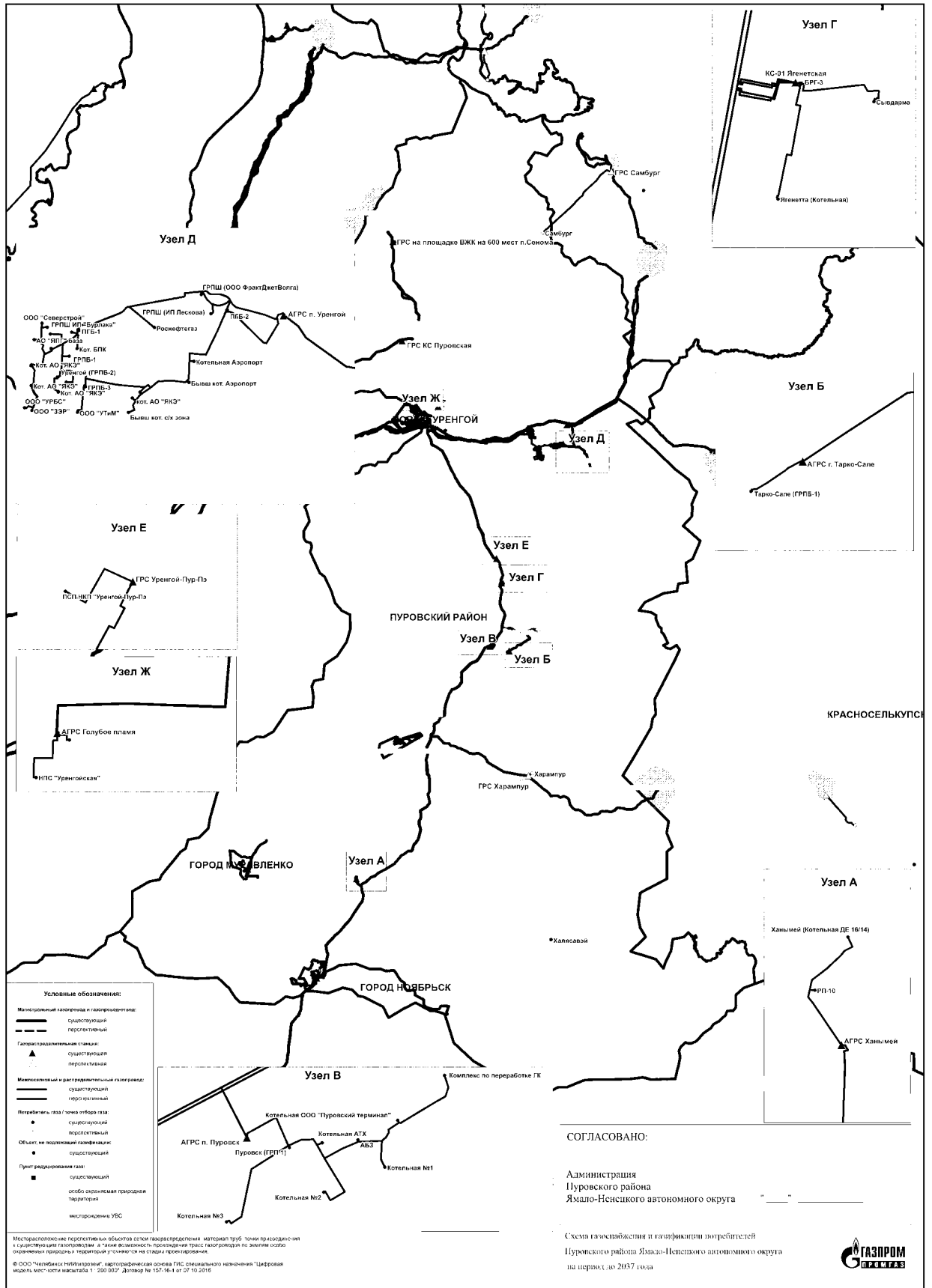
Схема газоснабжения и газификации потребителей Пуровского района Ямало-Ненецкого автономного округа на период до 2037 года
