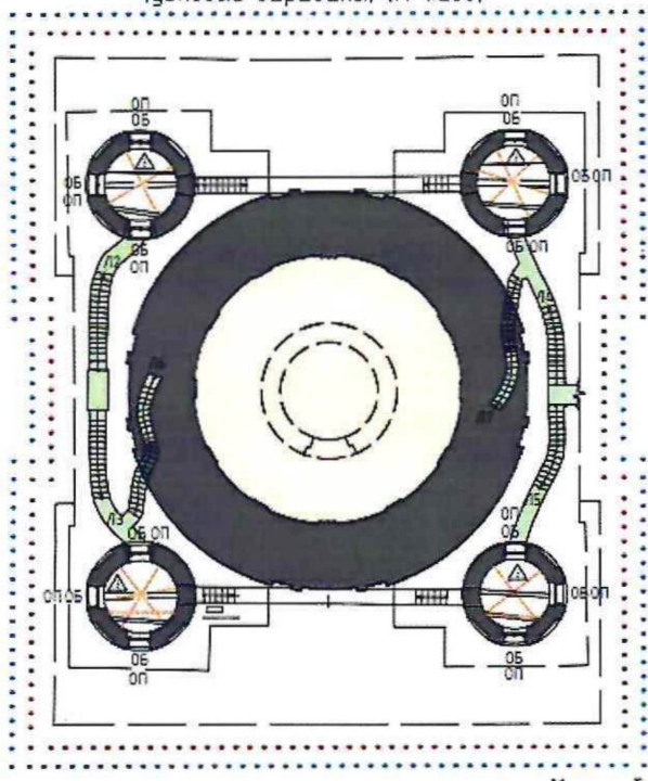
План на отметке +15,950 (узловые барабаны) (М 1:200)
