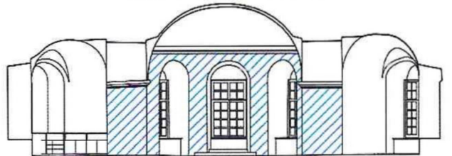
Развертка "Е-Е" (восточная стена)
