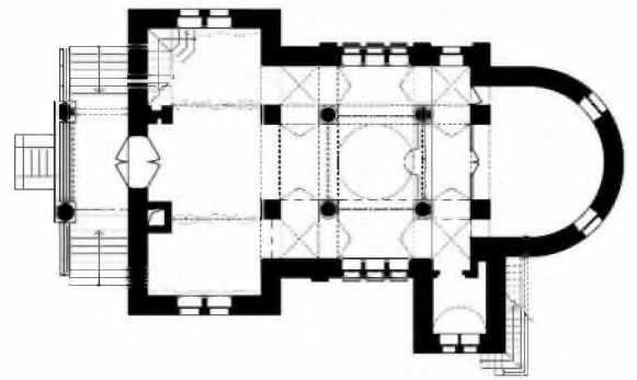
План – схема церкви
