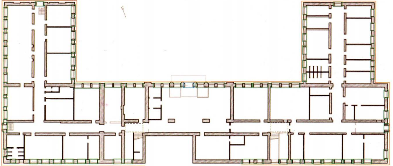
План первого этажа внутриквартального корпуса
