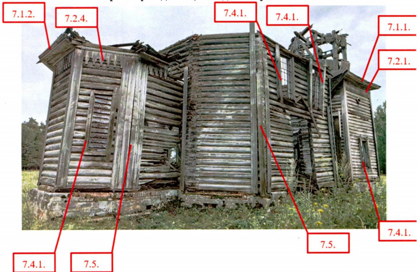
Северный фасад. Общий вид с северо-востока
