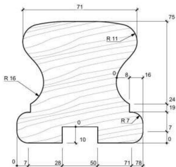
Шаблон 7. Деревянные перила парадной лестницы.
