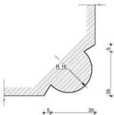
Шаблон 2. Оформление арочных проемов с коробовым завершением 1-го этажа.
