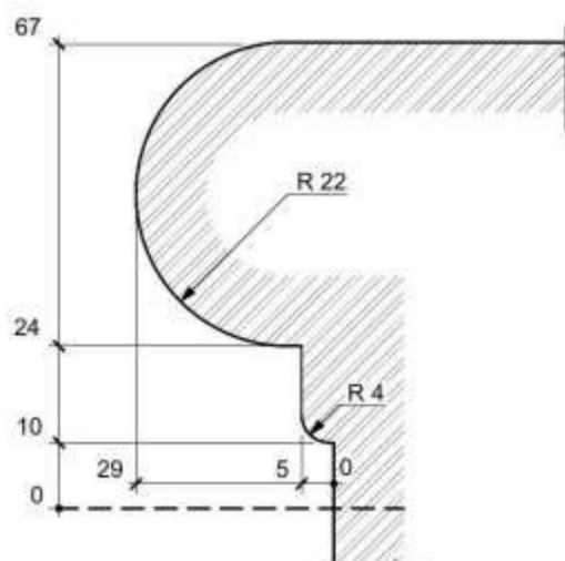
Шаблон 8. Каменная ступень.
