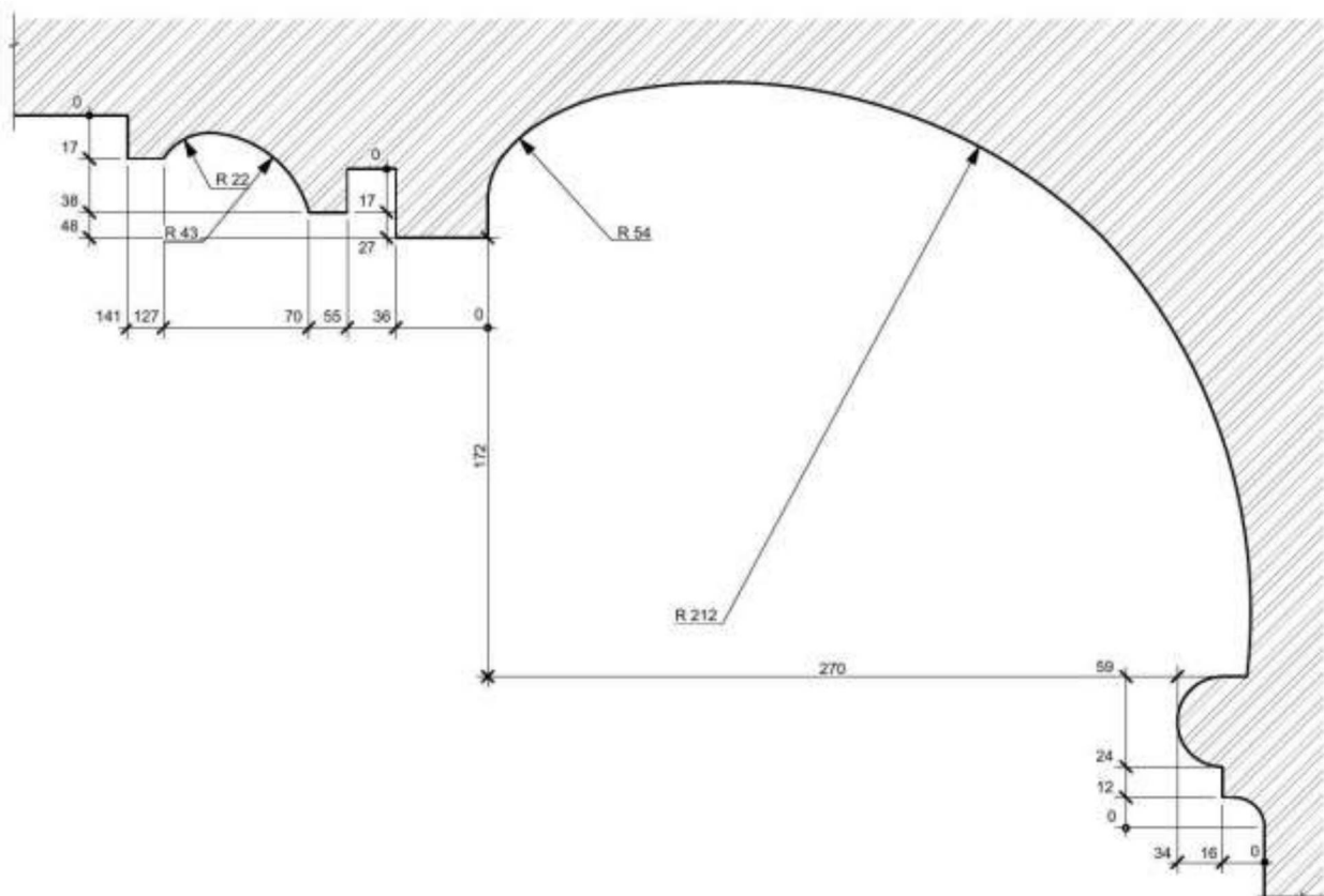
Шаблон 9. Шаблон потолочного карниза помещений 1-го и 2-го этажей.
