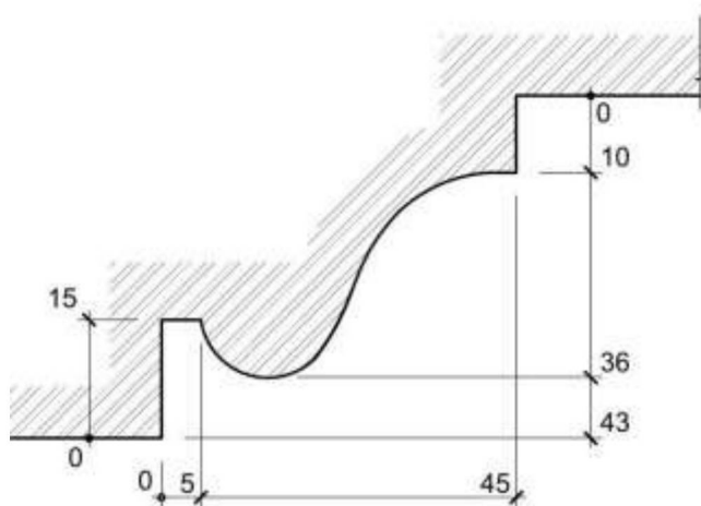
Шаблон 4. Тяга в оформлении нижнего подшива марша парадной лестницы.
