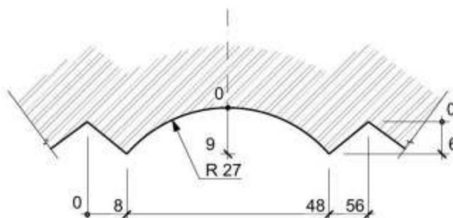
Шаблон 6. Тяга в оформлении внутренних углов крестовых сводов 1-го этажа.
