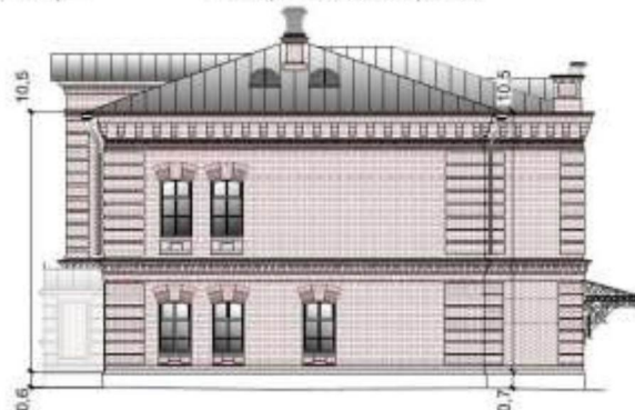
Северо-западный фасад
