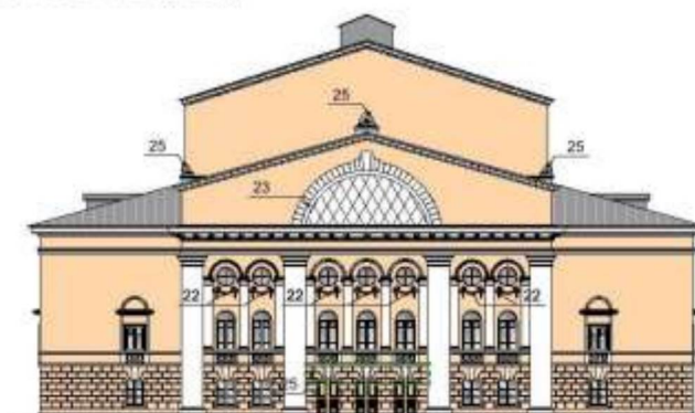
Юго-восточный фасад
