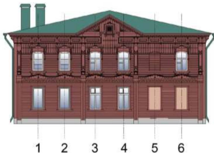
Северо-восточный фасад
