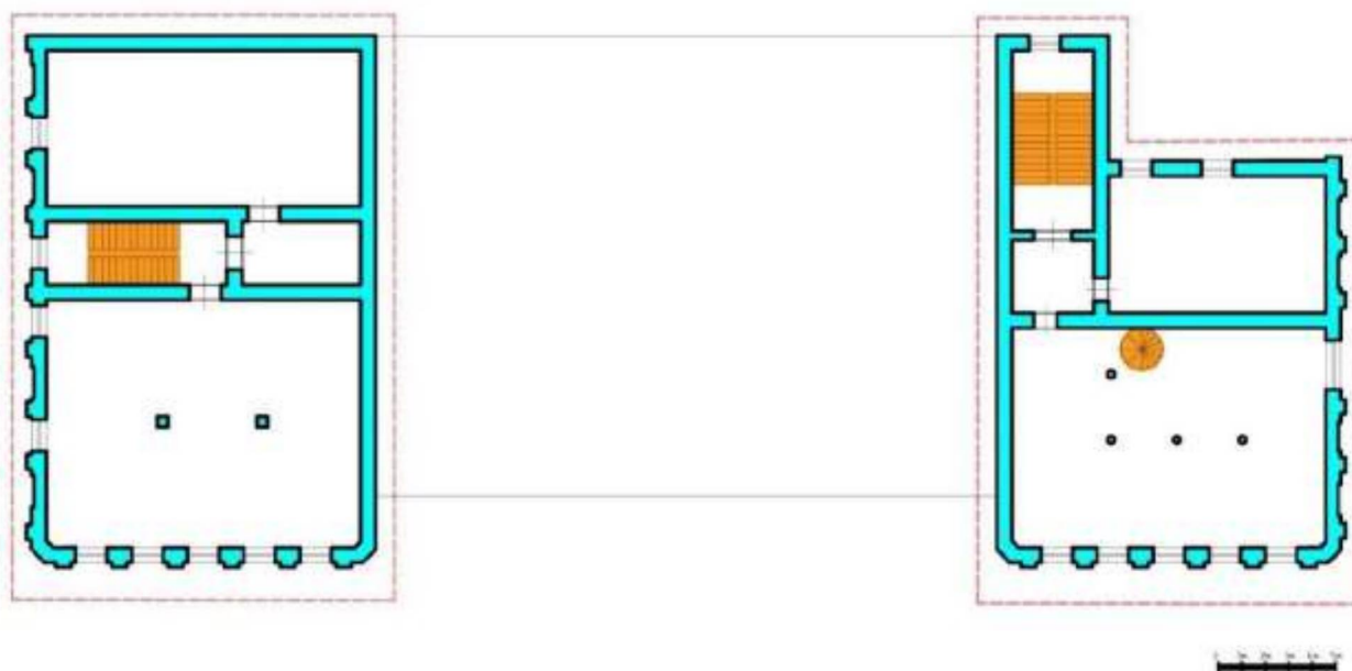
План 4 этажа
