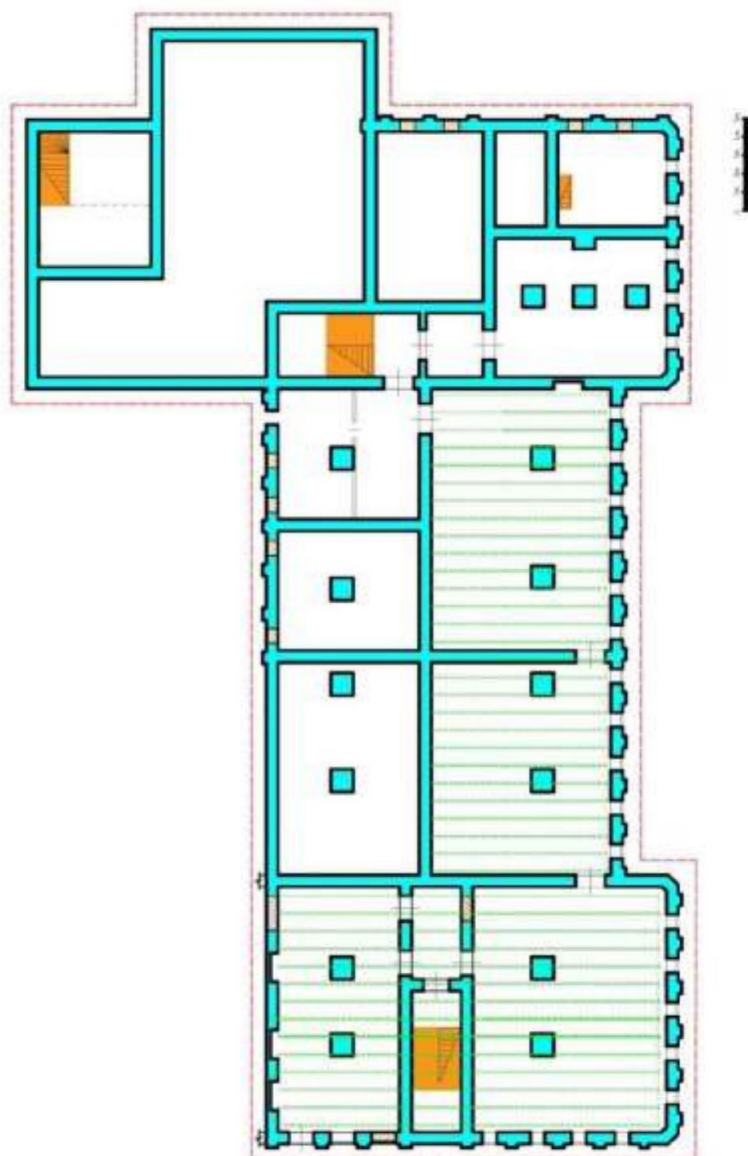
План подвала
