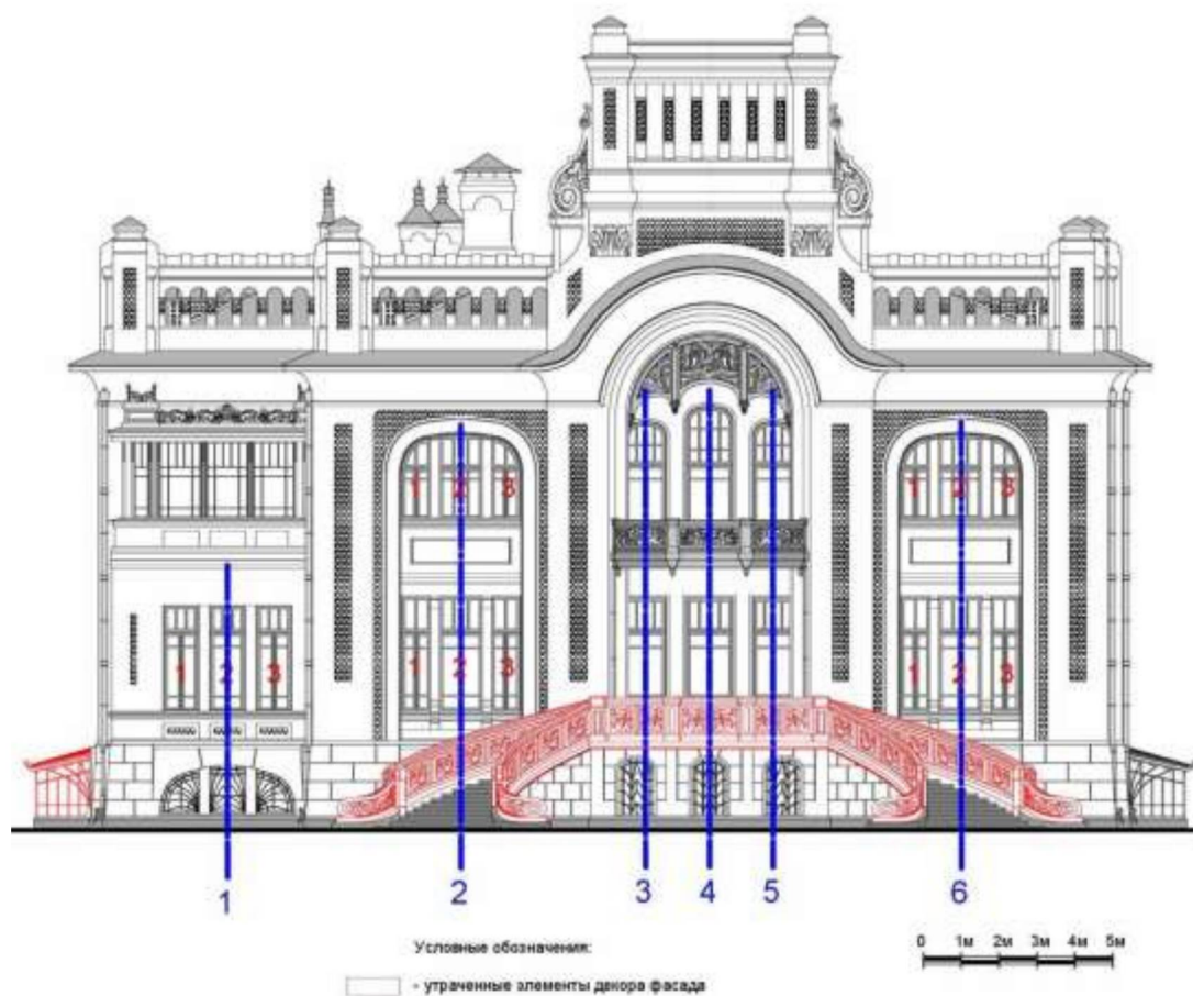
Северный фасад
