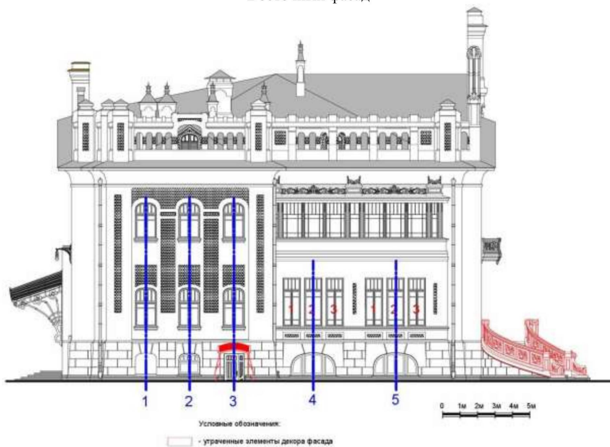
Северный фасад
