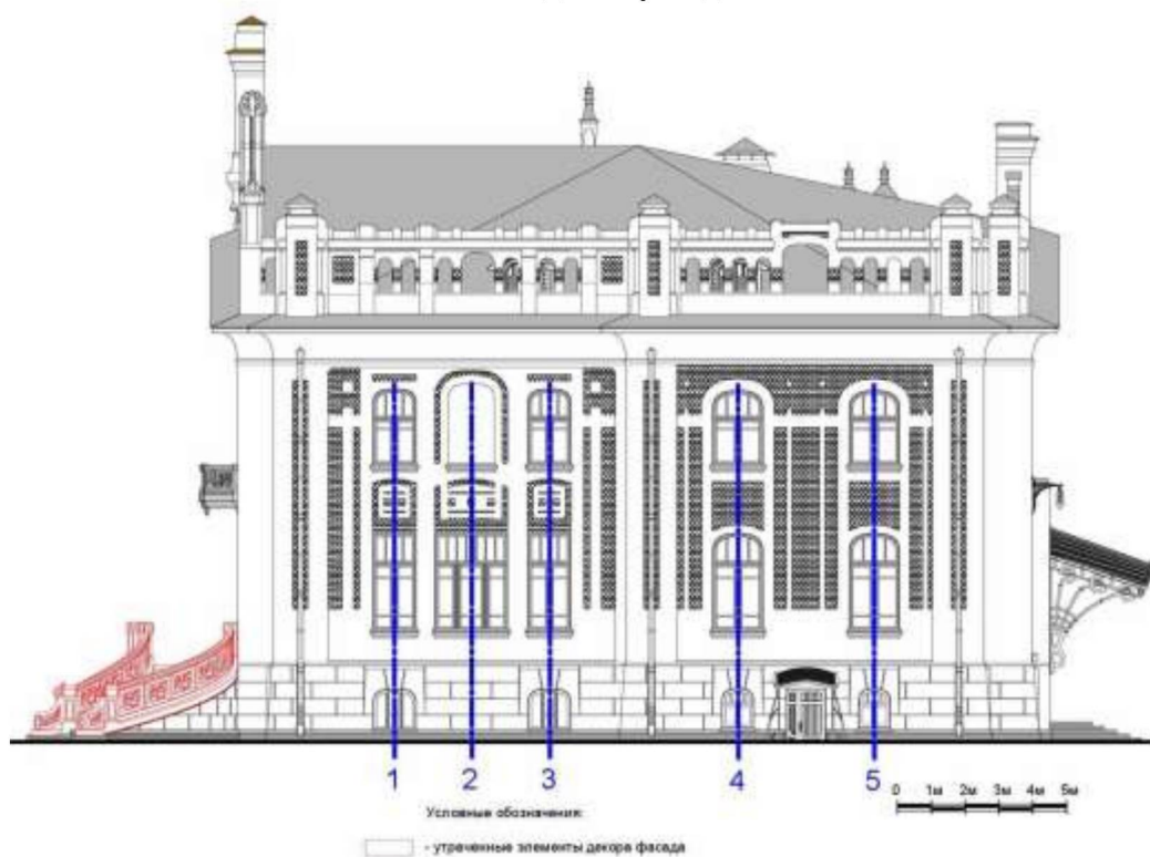
Западный фасад
