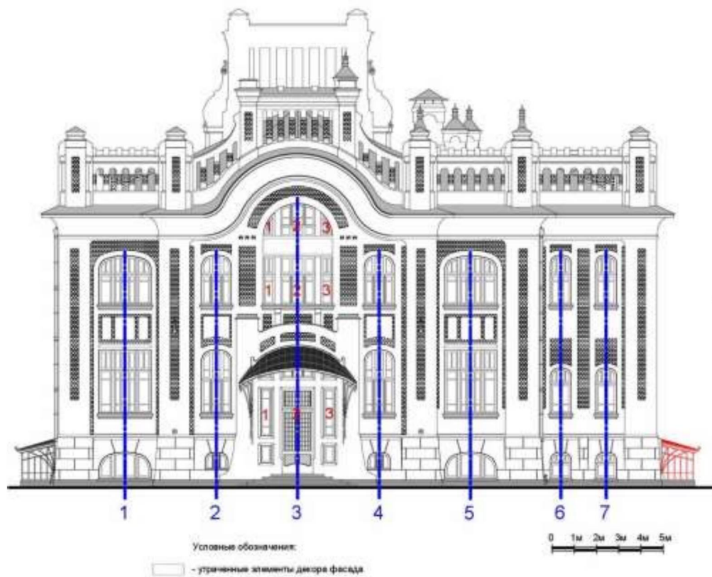
Западный фасад
