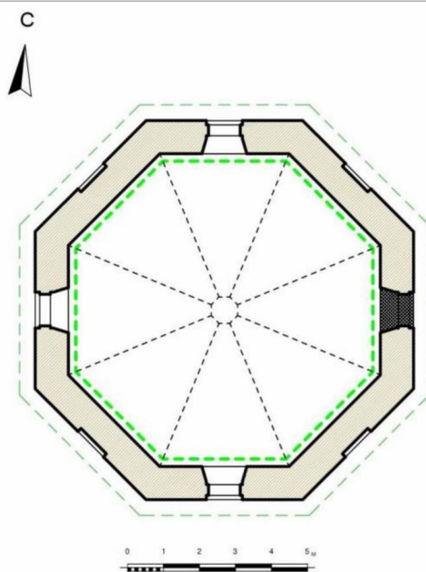
План восьмерика
