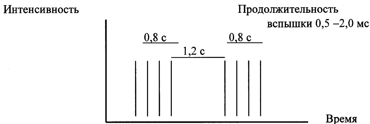
Рисунок 1. Характеристики вспышек вертодромного маяка.
