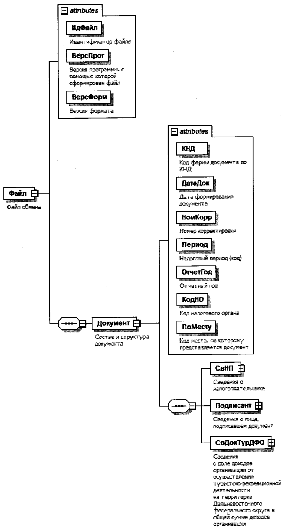
Рисунок 1. Диаграмма структуры файла обмена
